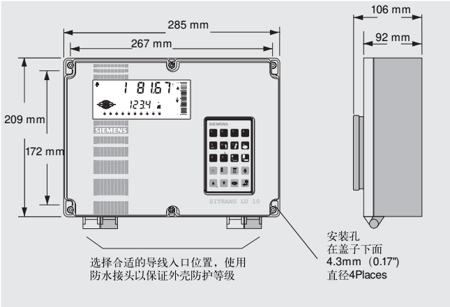
SITRANS LU 10 尺寸
