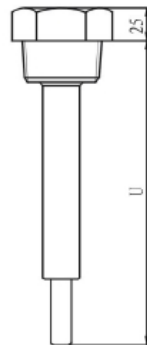
22型温度套管
